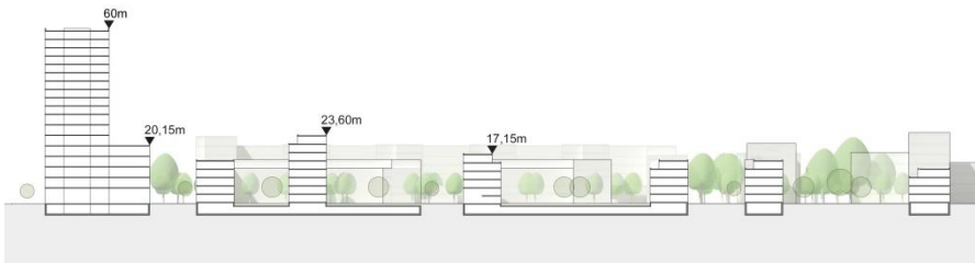
Schnitt 2-2
